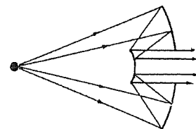
Figure 4. Le paragraphe 5 correspond à des systèmes d'éclairage. On remarquera que Mersenne décrit les montages proposés en suivant le sens de la lumière.
